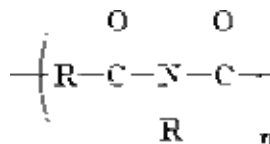
linear polyimide
